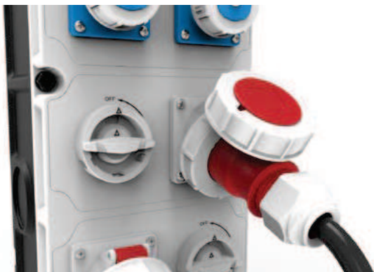
Detail van de afschakelbaar/vergrendelbaar flensplaat.
